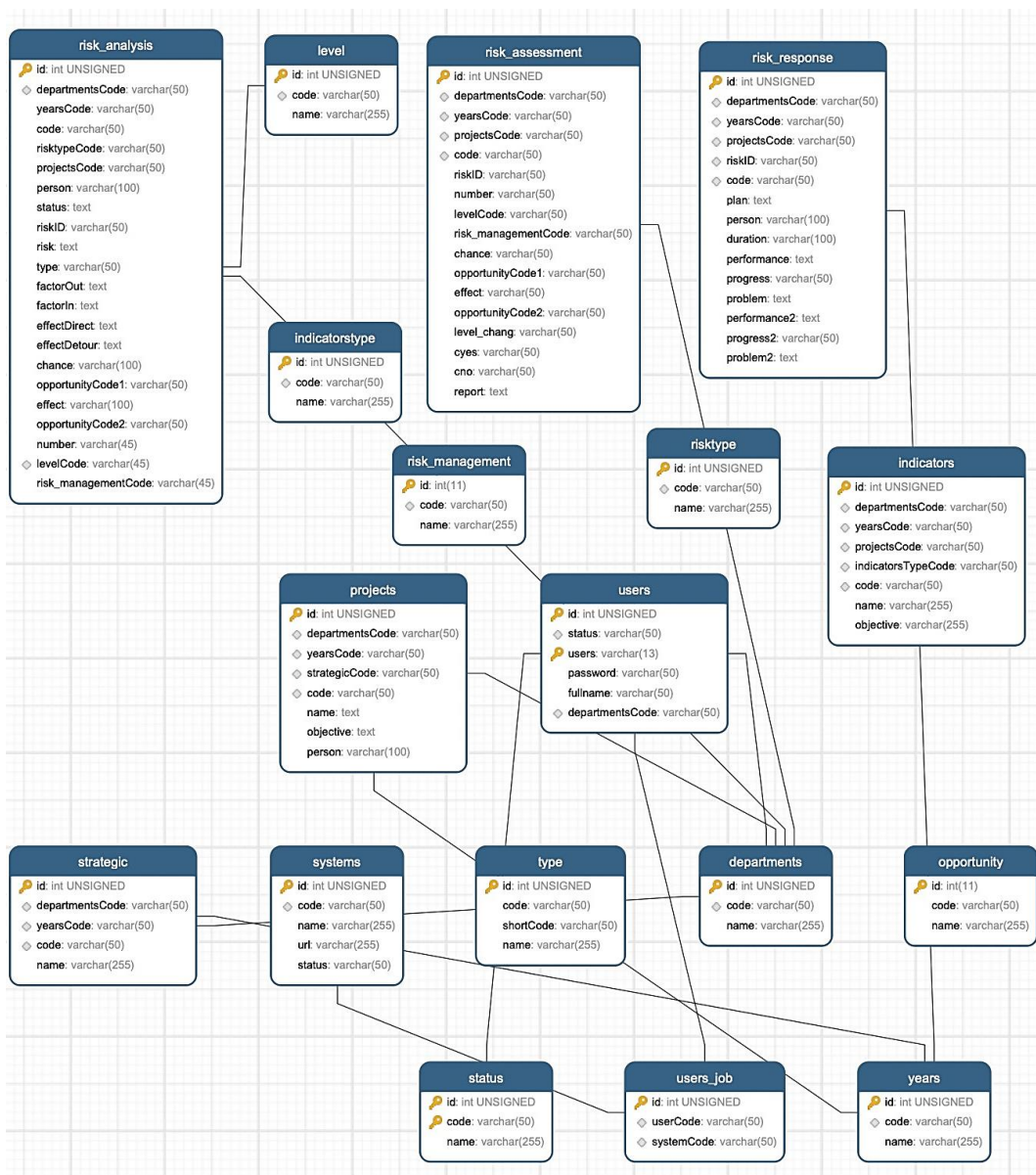
ภาพที่ 2 แผนภาพอีอาร์ (ER diagram) แสดงการออกแบบฐานข้อมูลของระบบ
